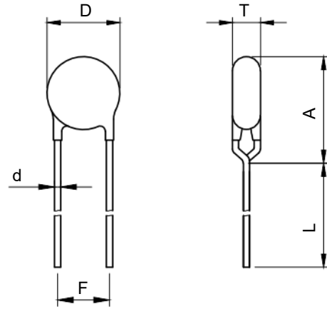
Y型引线 Inline Crimp Lead
