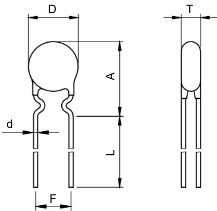
内弯型引线 Inward Crimp Lead
